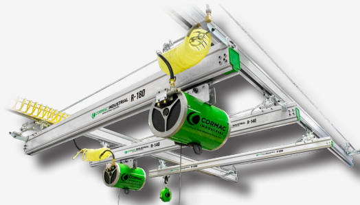
Gruas puente
